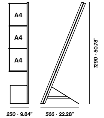
IFT Triple · Triple
