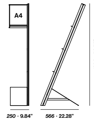
IFS Simple with shelf · Simple con repisa
