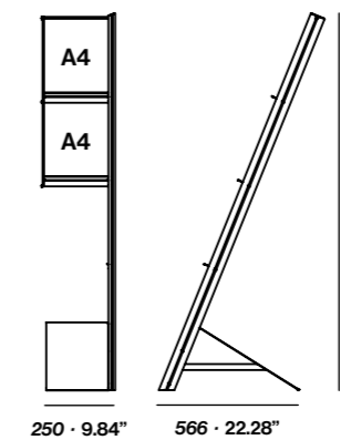
IFD Double with shelf · Doble con repisa
