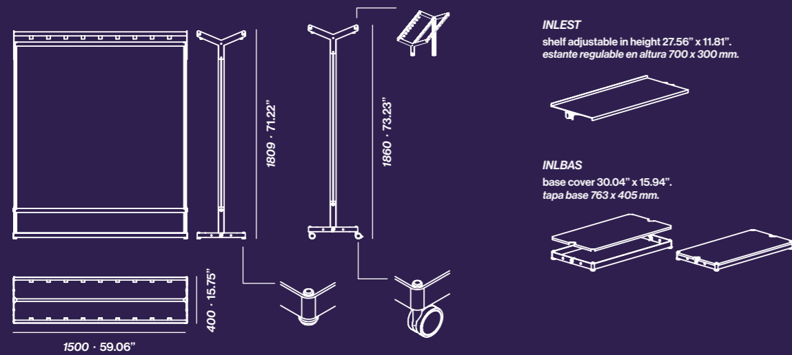
INLD15PF adjustable feet · pies regulables INLD15RD wheels · ruedas INLIN 758 accessories · accesorios
